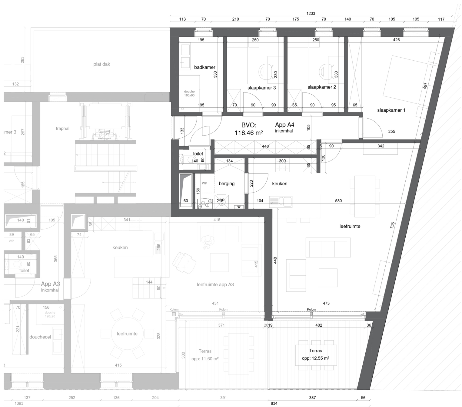
Grondplan
